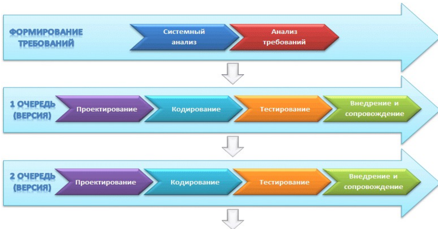
Рис.3.2. Инкрементная стратегия
